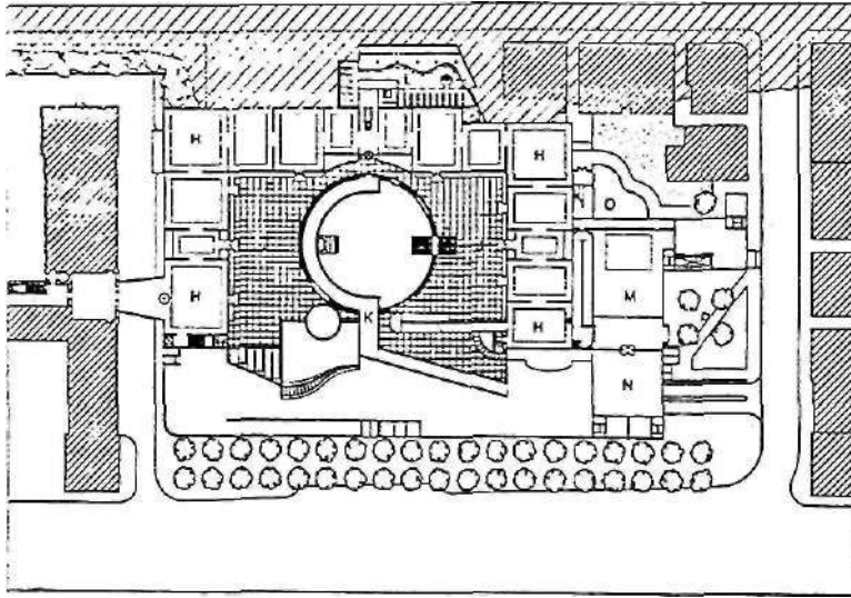
Jamo Slirling, Ampliación de la Staatgalerie de Stuttgart, plantas.
